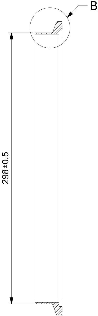
SECTION A-A
