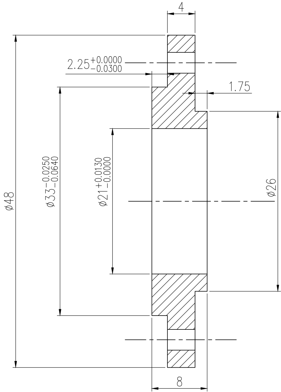
SECTION A-A
