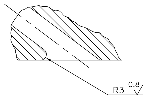
DETAIL-D SCALE-1:1
