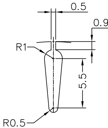
DETAIL- 'A'
