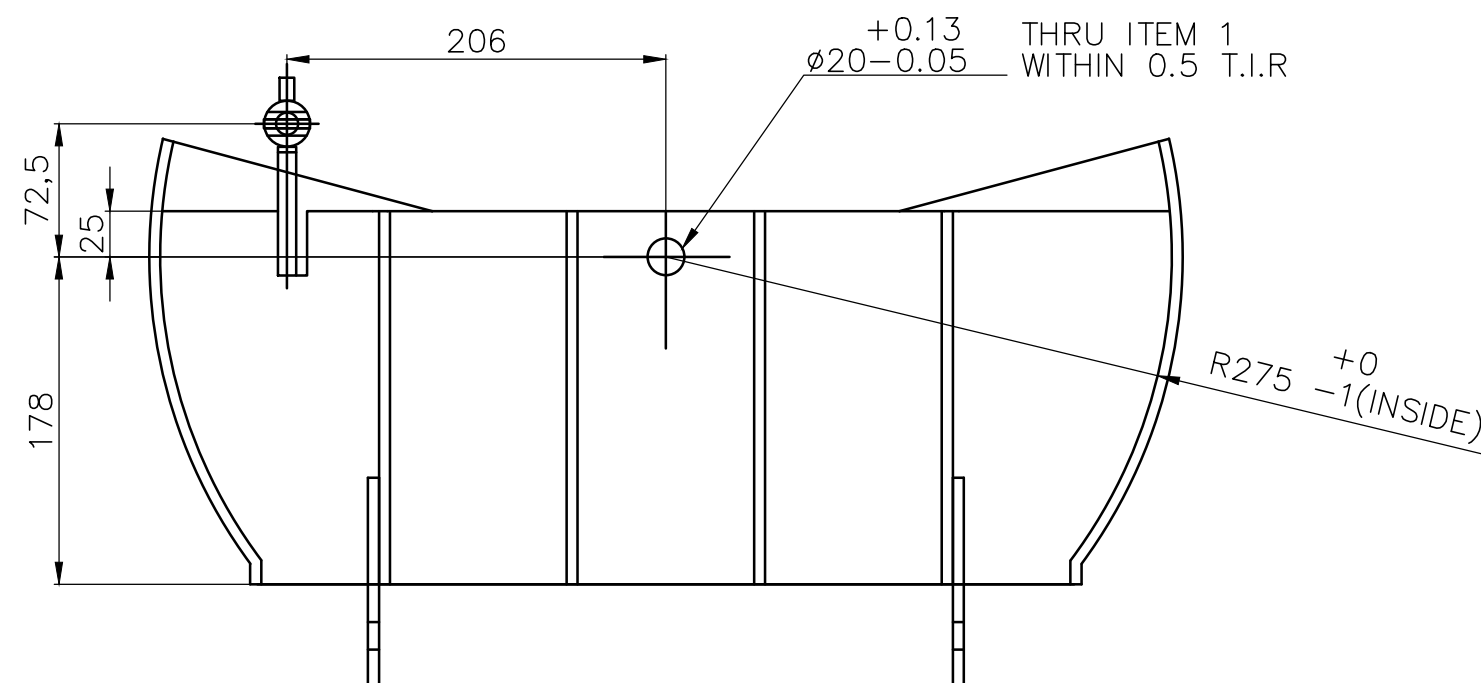
SECTION A-A SCALE 1:4
