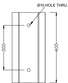
400x110 DOOR DETAIL
