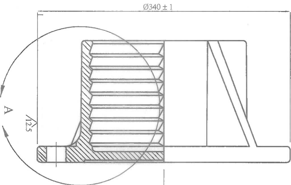
SECTION 'B-B'
