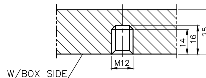
C-C SCALE 1:1
