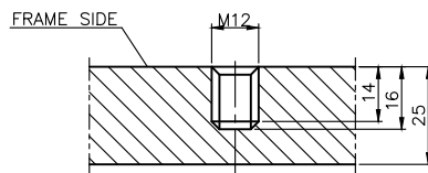
B-B SCALE 1:1
