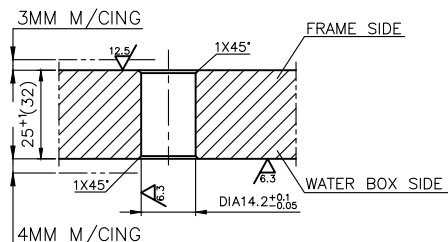
A-A SCALE 1:1
