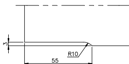
DETAIL — II SCALE 1:1
