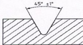
a) Type A Radius of notch tip r_N = (0,25 \pm 0,05) mm
