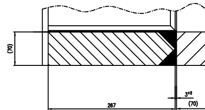
SECTION-BB SCALE: -1:2.5
