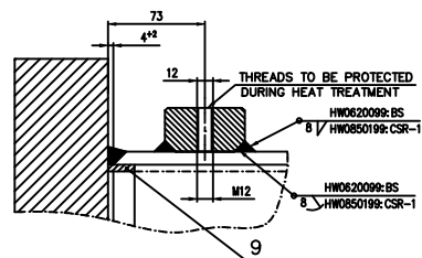
VIEW-A SCALE:-1:2
