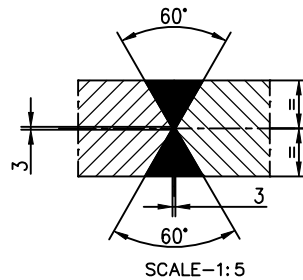
SCALE-1:5
