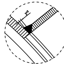
DETAIL-I SCALE:-1:1
