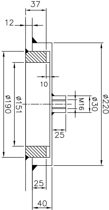
Detail-B
