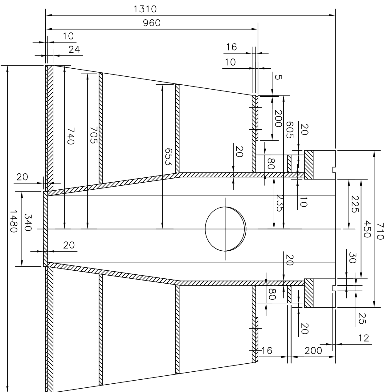
SECTION D-D
