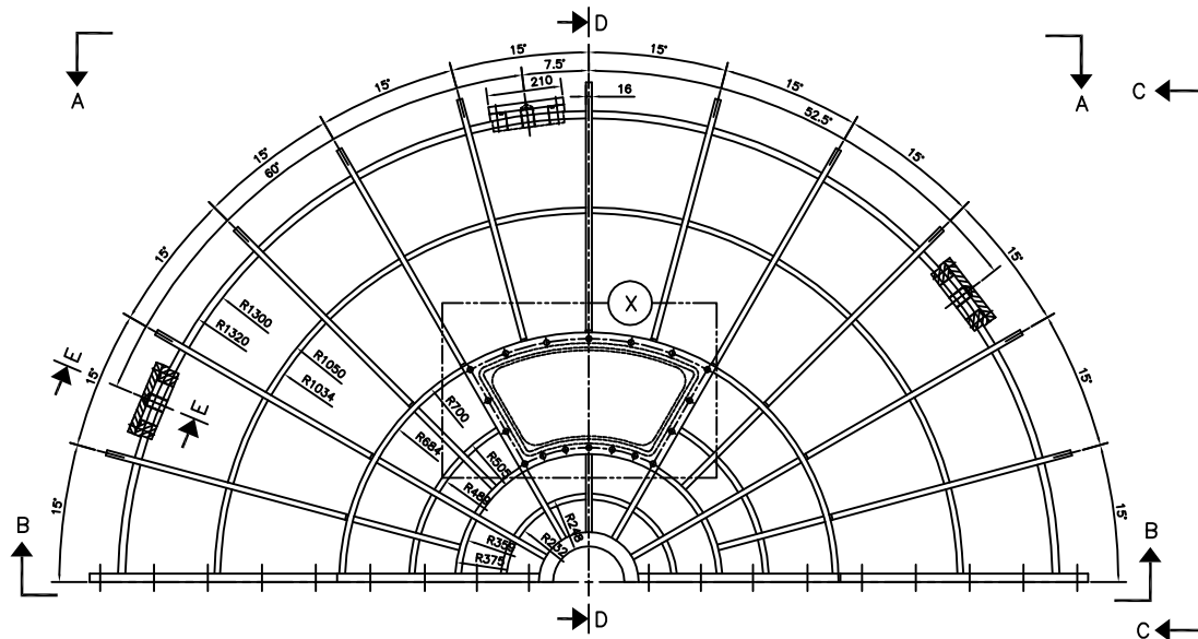
TOP VIEW A-A
