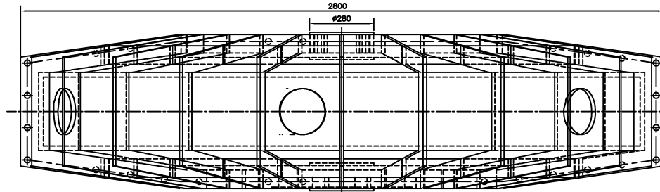
TOP VIEW A-A
