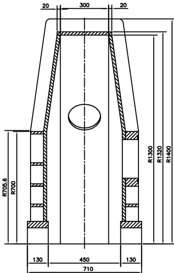
SECTION D-D
