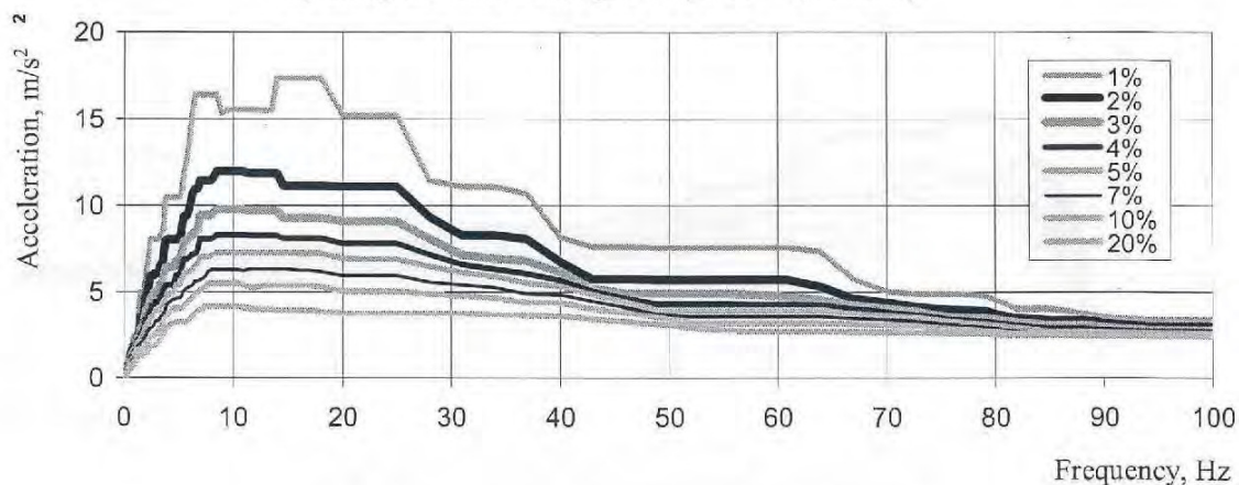
b) along the horizontal grid y (ZPA = 2,33 m/s 2 )
