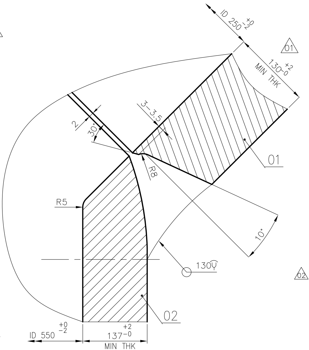
DETAIL-B
