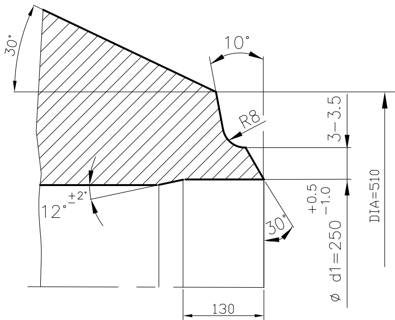
DETAIL-D
