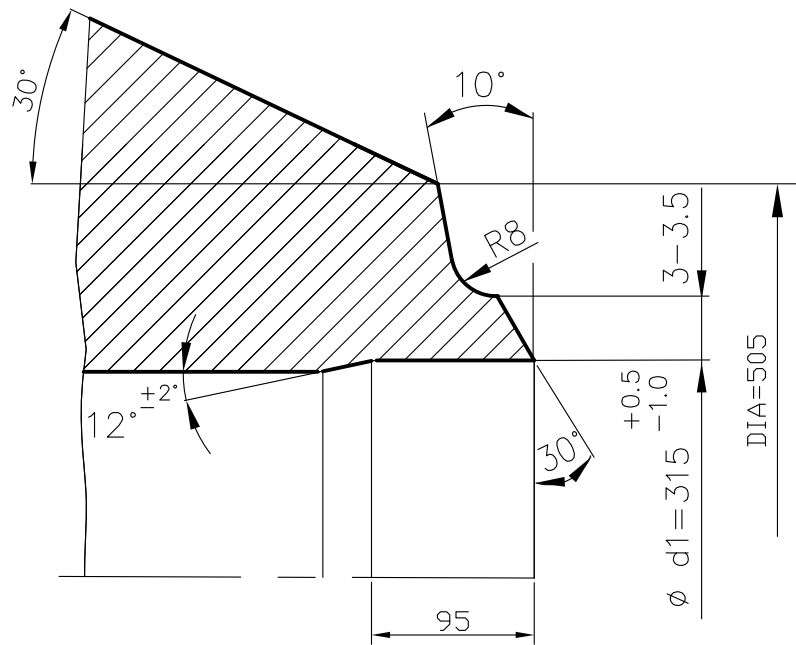
DETAIL-E
