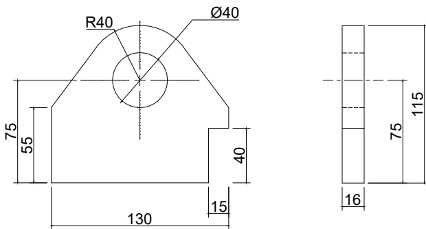
LUG DETAIL
