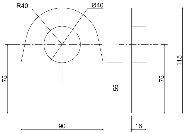
LUG DETAIL
