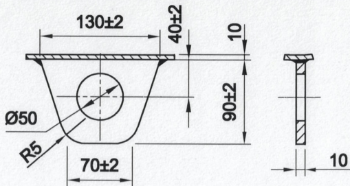
LUG DET.-S
