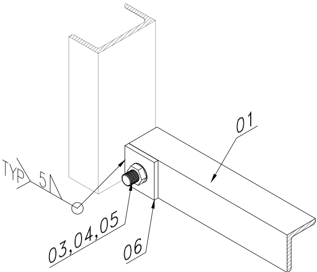
DETAIL- 'X' (TYP)
