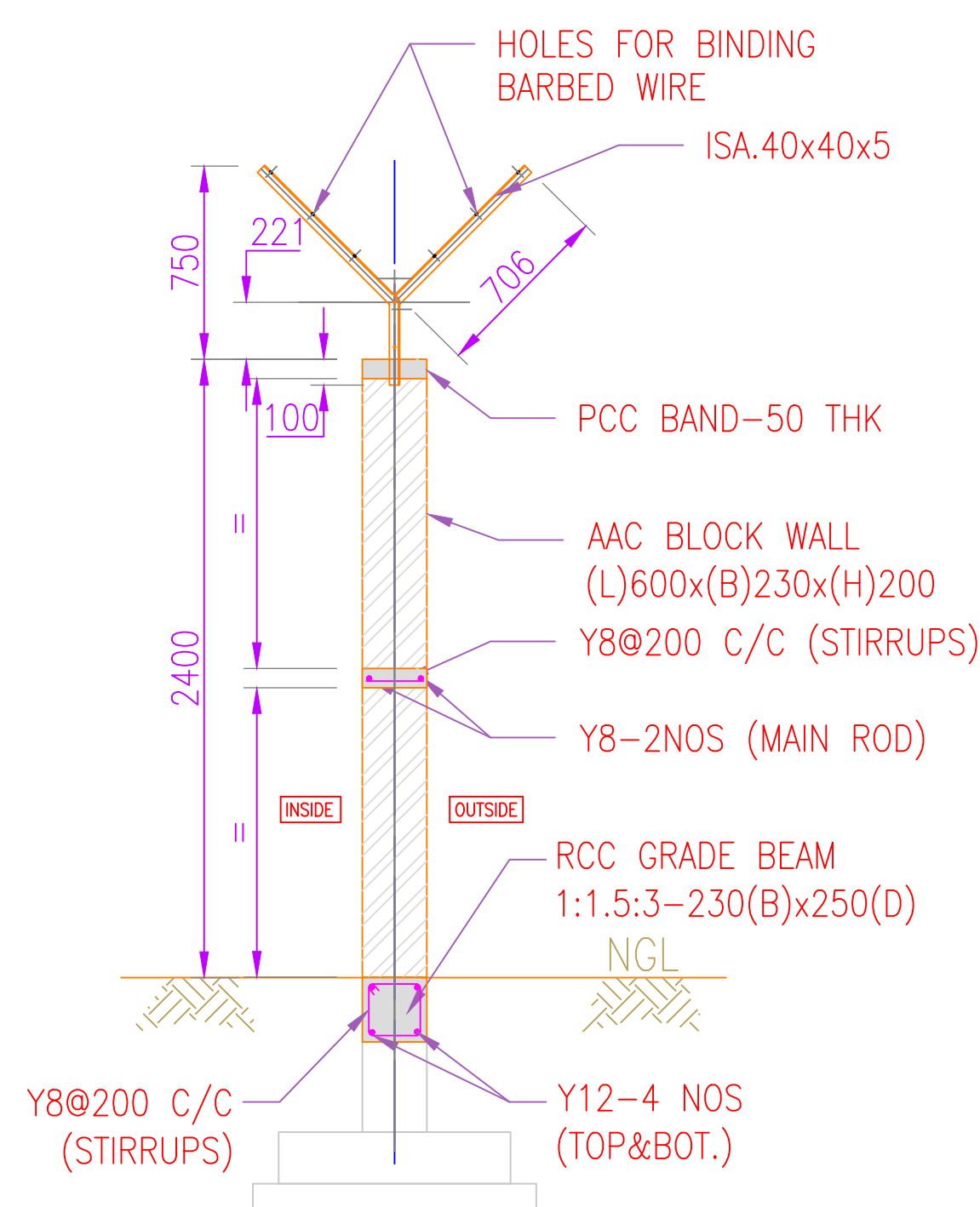
SECTION B-B (TYP.)
