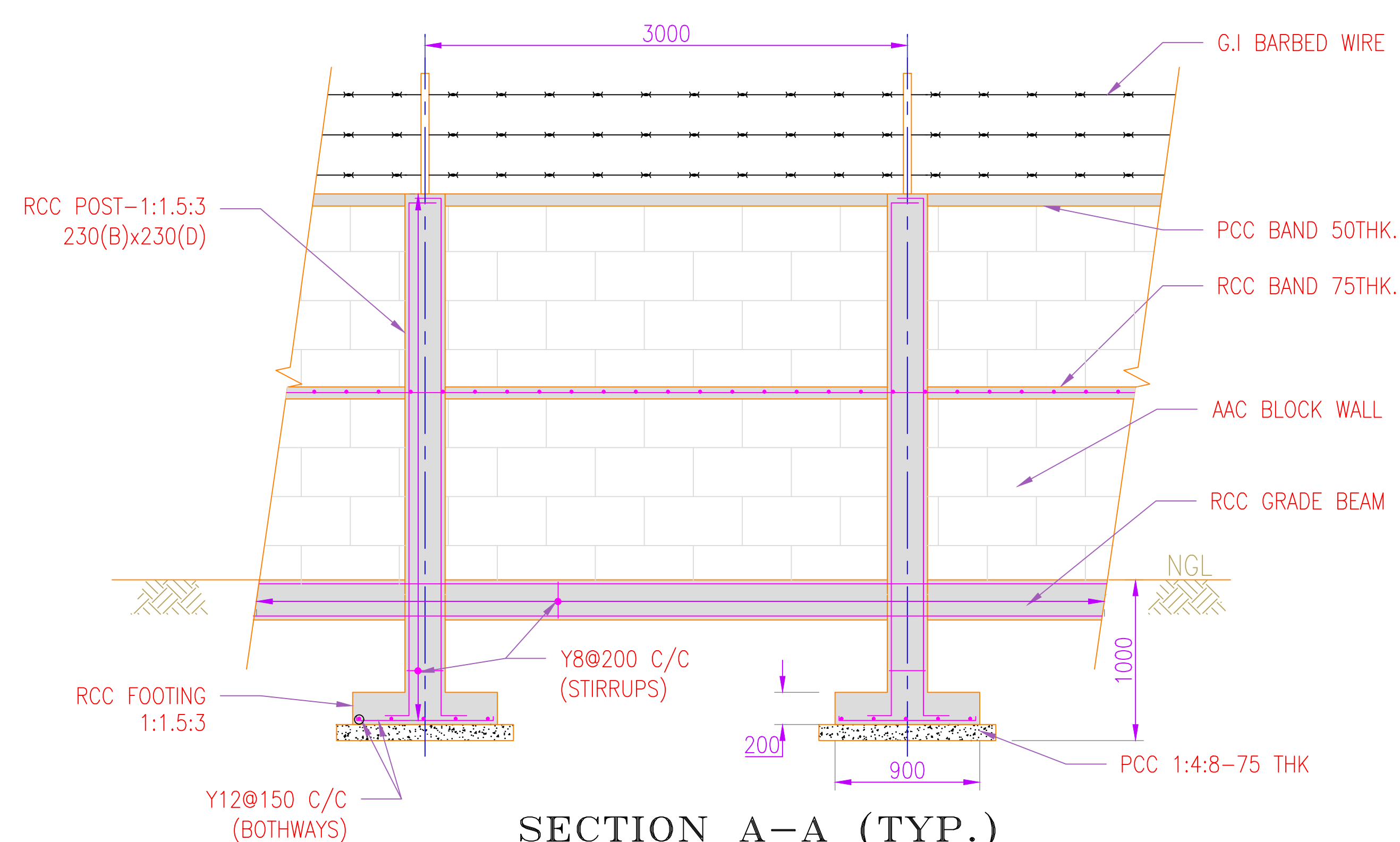
SECTION A-A (TYP.)
