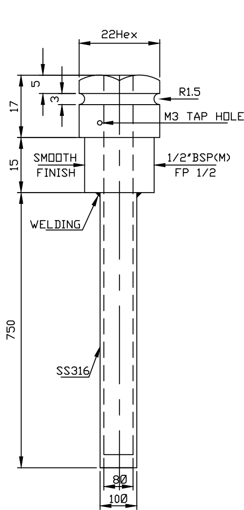
THERMOWELL
