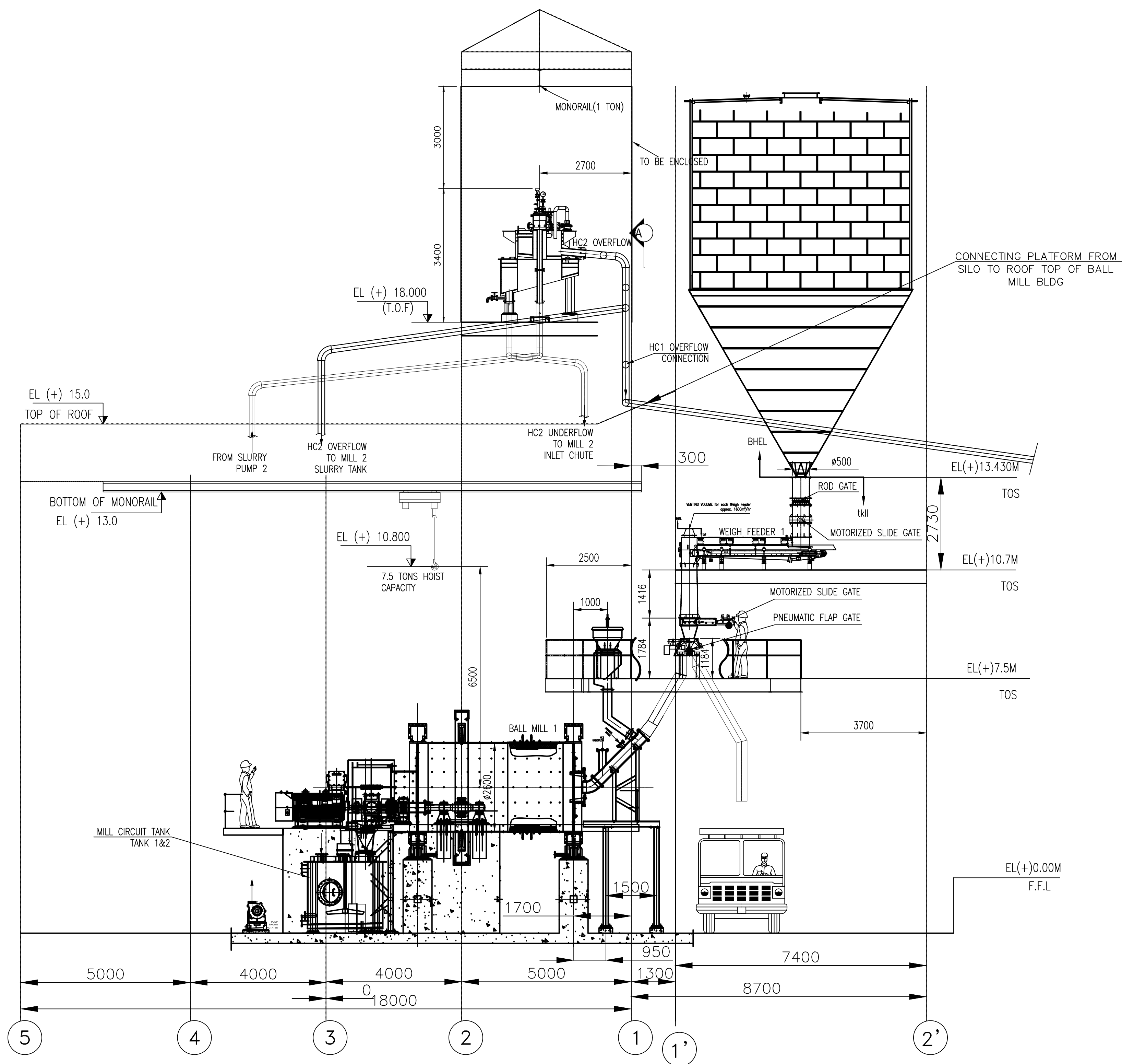
ELEVATION
