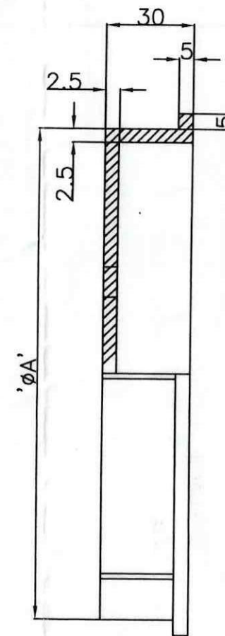
SECTION A-A
