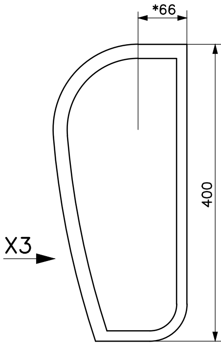
ITEM-04 (1:5)
