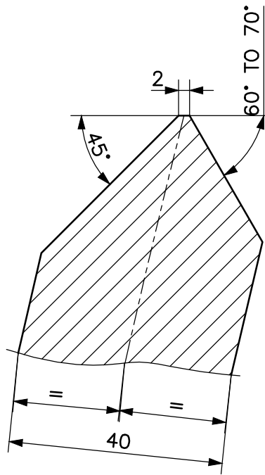
ITEM-04 (1:5)
