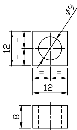
ITEM - 015 (SCALE-1:1)
