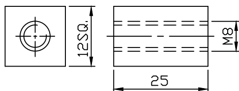
ITEM - 018 (SCALE-1:1)
