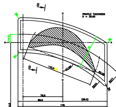
SECTION A9-A9
