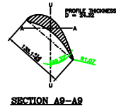
SECTION A9-A9
