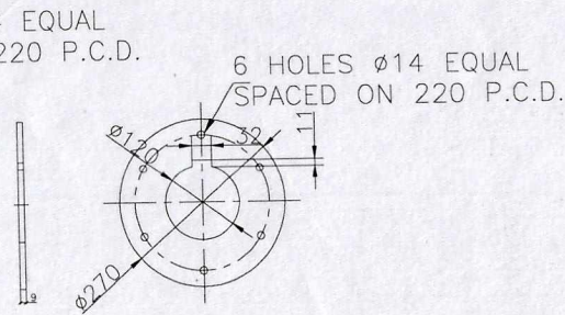
SPACER 9 TK QTY. 02 (IT.004)
