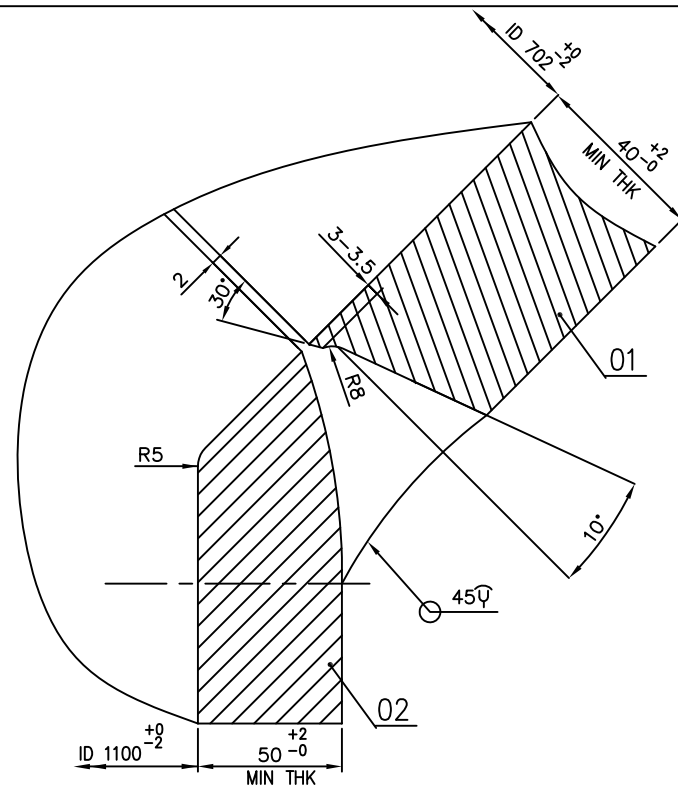
DETAIL-B
