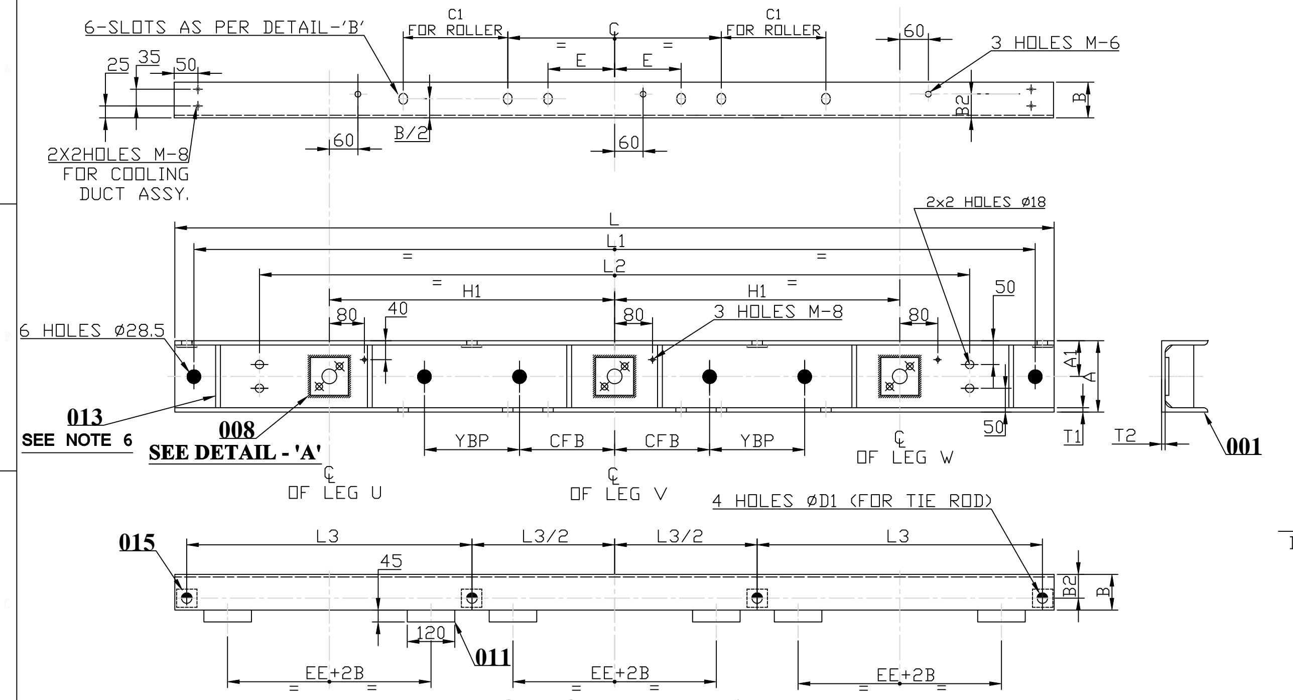
H.V. BOTTOM END FRAME
