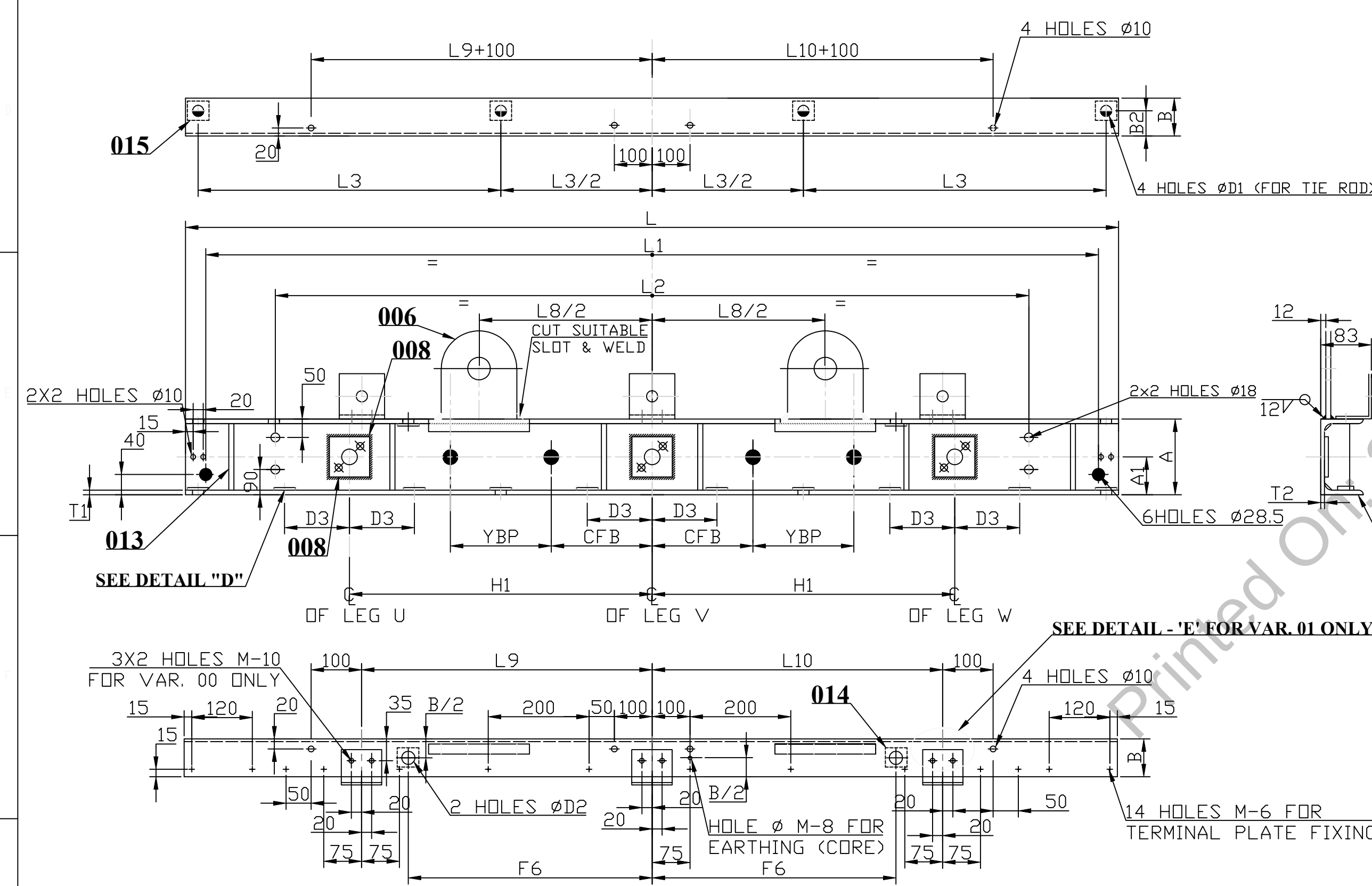
H.V. TOP END FRAME
