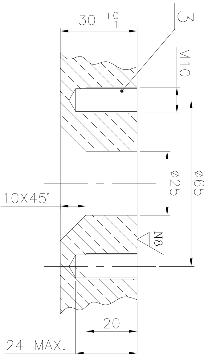
DETAIL: B-B
