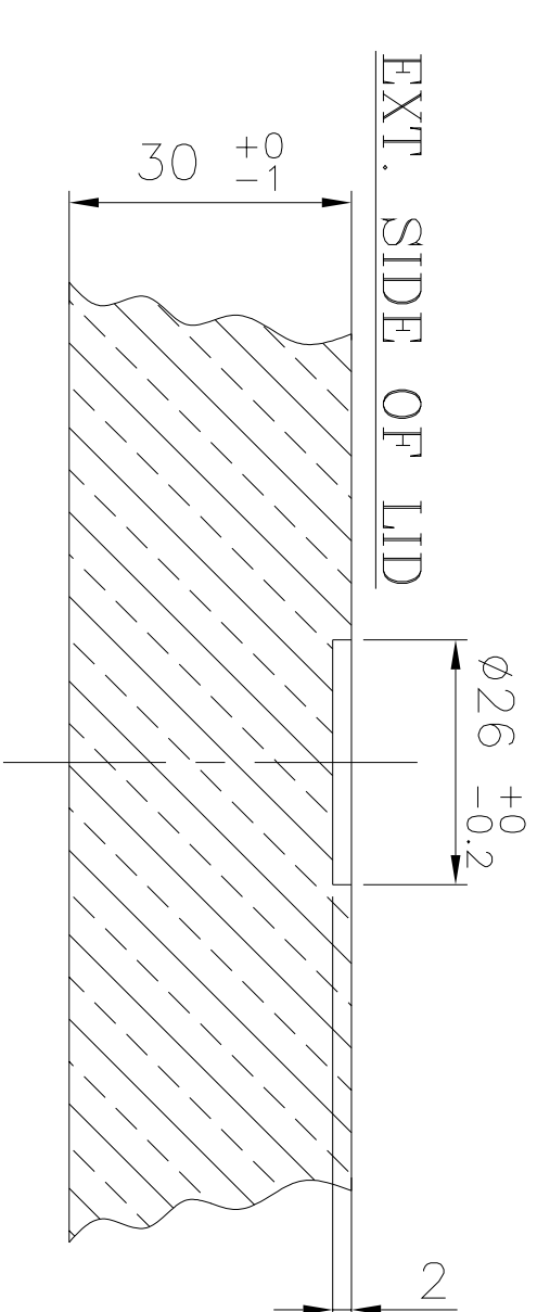
DETAIL: E-E
