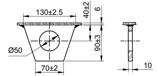
LUG DET.-S WT.-0.55 Kg (Approx.)
